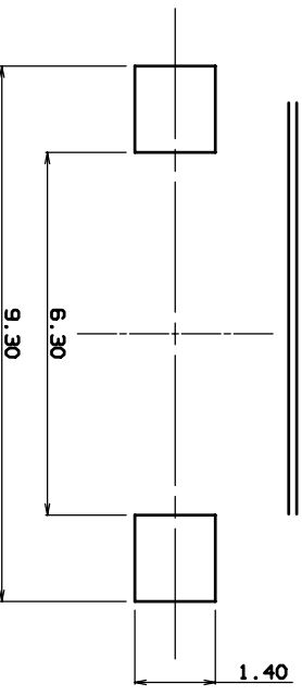
P.C.B LAND DIMENSION
