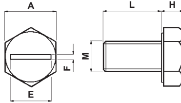
VITI A TESTA ESAGONALE. HEXAGONAL HEAD SCREWS.
