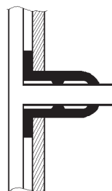
Tipo 3 Type 3
